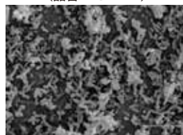
菌体の電子顕微鏡画像 (品番: LBEV-R2)
